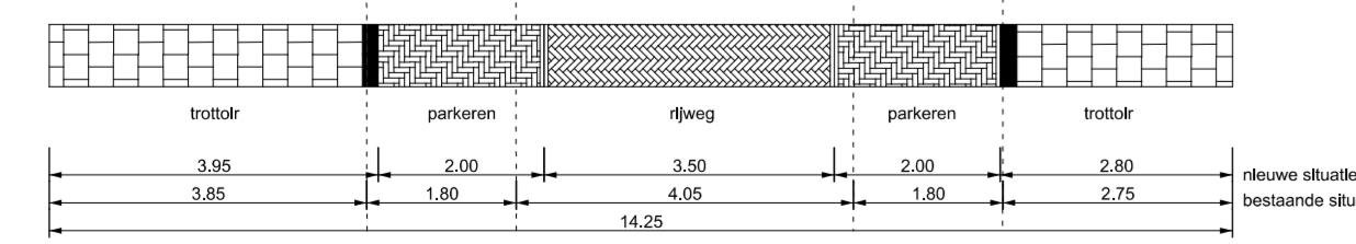
profiel 1:100 MERKUSSTRAAT PROFIEL: RIJBAAN 3.50 METER
